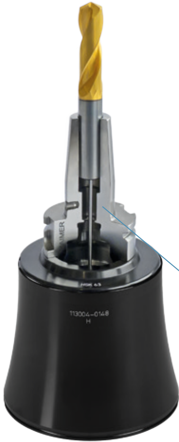
Resim: Altlık ile birlikte Quick Set (Altlık paket içerisinde dahil değildir) Picture shows: Quick Set with base holder (Base holder not included in delivery)
